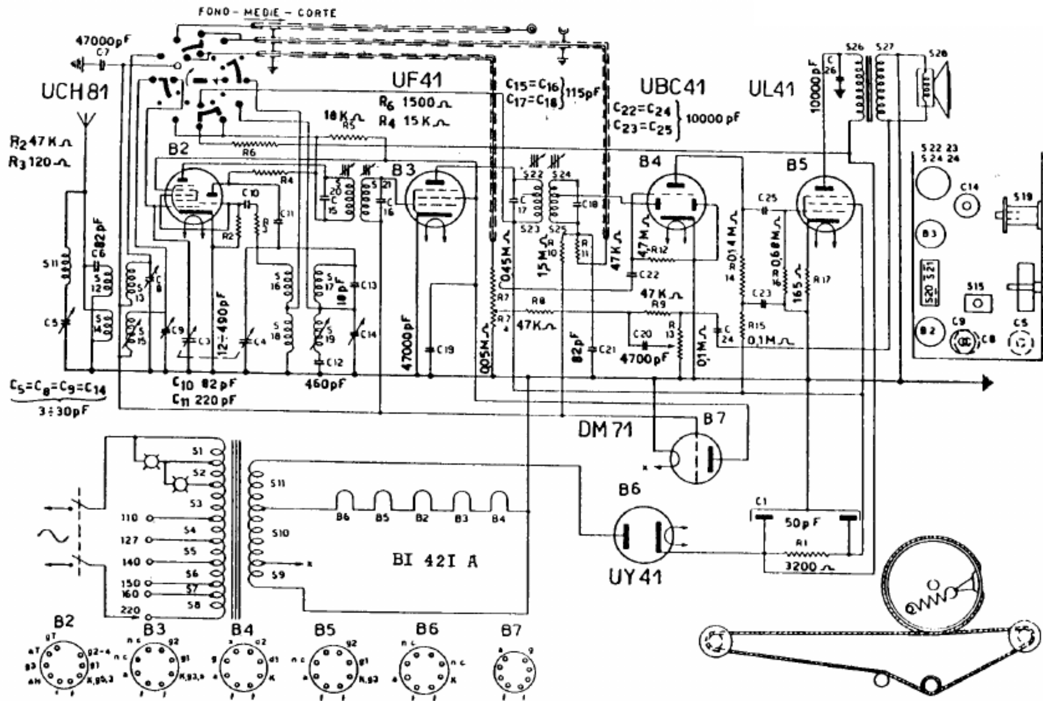
PHILIPS RADIO - Mod. B. 421 A. Una gamma onde medie da 184 a 545 m ed una ad onde corte da 16,5 a 50 m. Mixer-Neval. Media frequenza 468 kc/s. Corrente anodica totale 75 mA. Consumo 43 watt.
